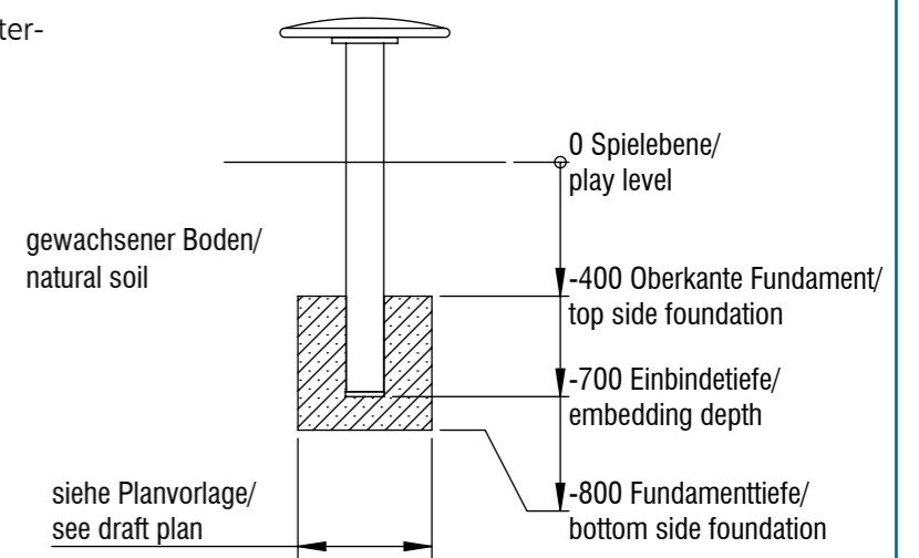
Fundamentalschnitt Großer Käfer/ foundation cut big beetle FS13 - FS14
