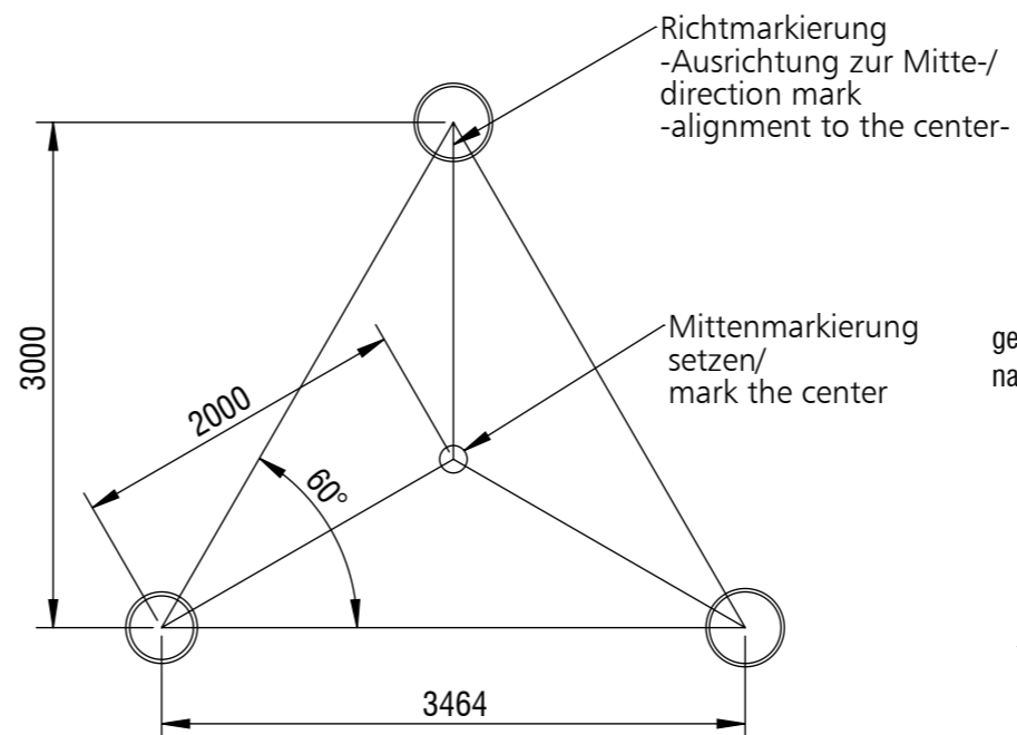
Fundamentalschnitt Großer Käfer/ foundation cut big beetle FS13 - FS14
