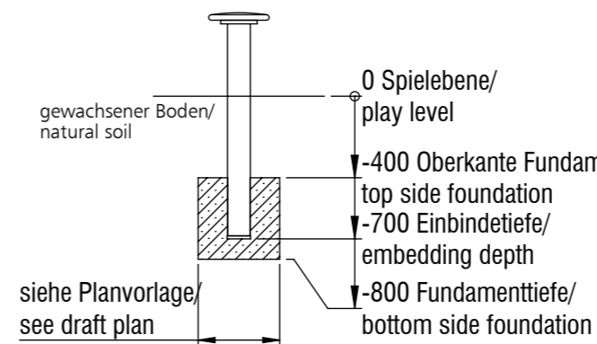
Fundamentalschnitt Kleiner Käfer/ foundation cut small beetle FS07 - FS12
