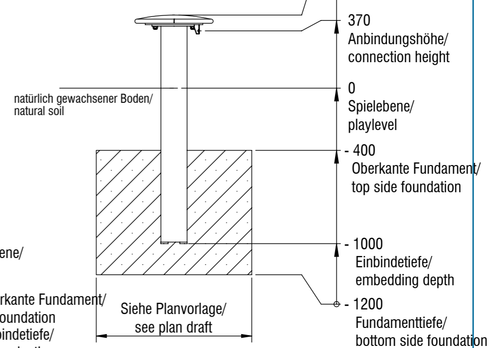
Fundamentalschnitt Flanschsäule/ foundation cut flange posts FS01 - FS06
