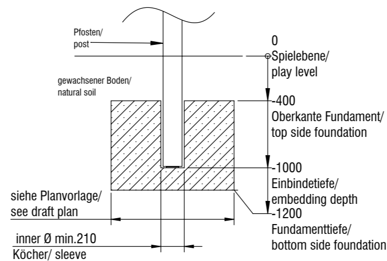
Fundamentalschnitt Pfosten/ foundation cut SP01 - SP09
