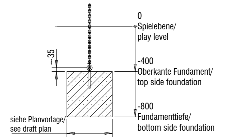
Fundamentalschnitt Lianenpark/ foundation cut liana park
