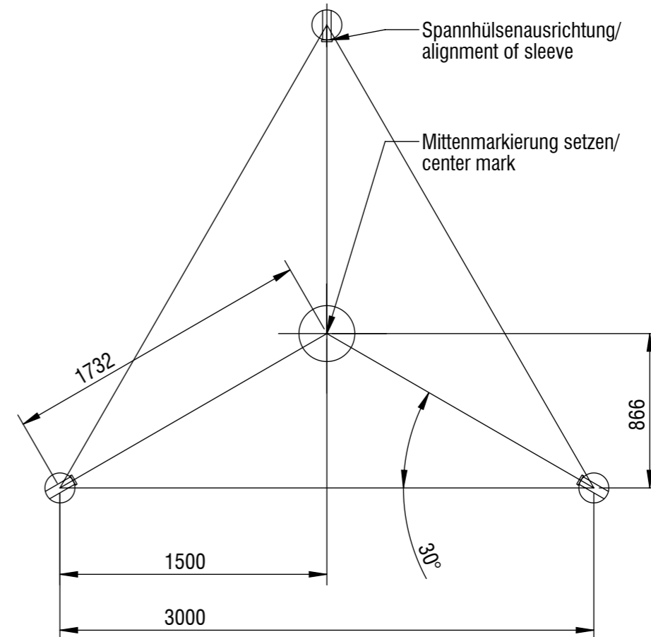
Ausrichtung der Pfosten/ Alignment of posts SP02, SP04, SP05
