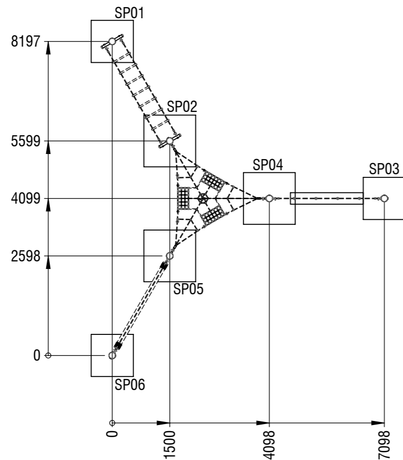
Fundamentgrößen foundation sizes
